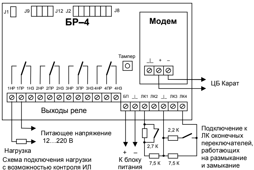
Рис. 1 Схема внешних соединений блока реле «БР-4»
